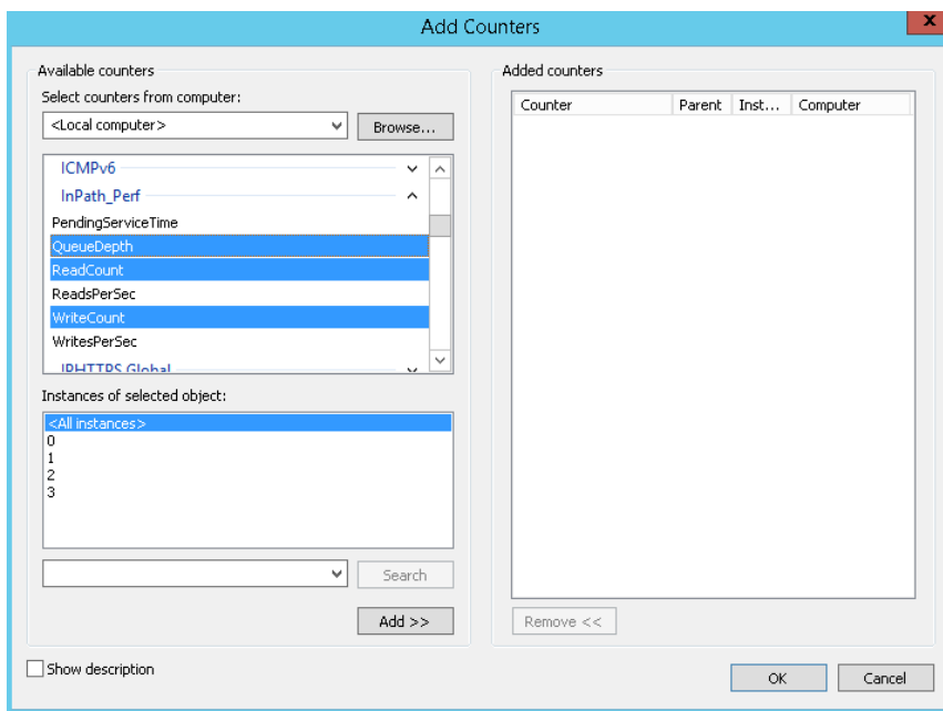
图 4-23 选择要查看的监控项
