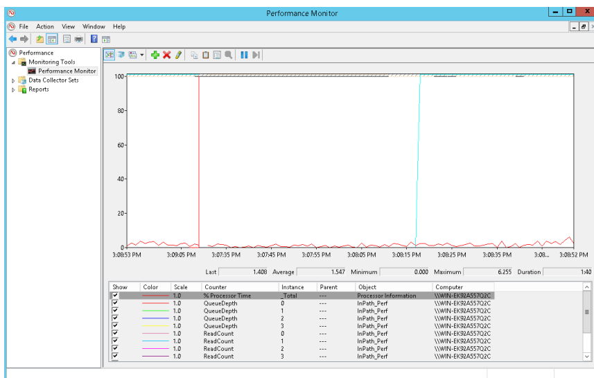
图 4-24 按路径画出的监控线图
