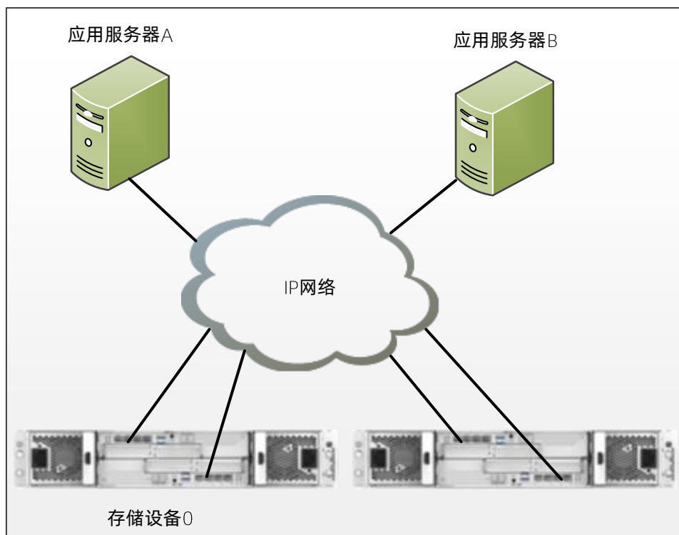
图 1-4 采用 IP 网络连接应用服务器与存储设备的组网方式
