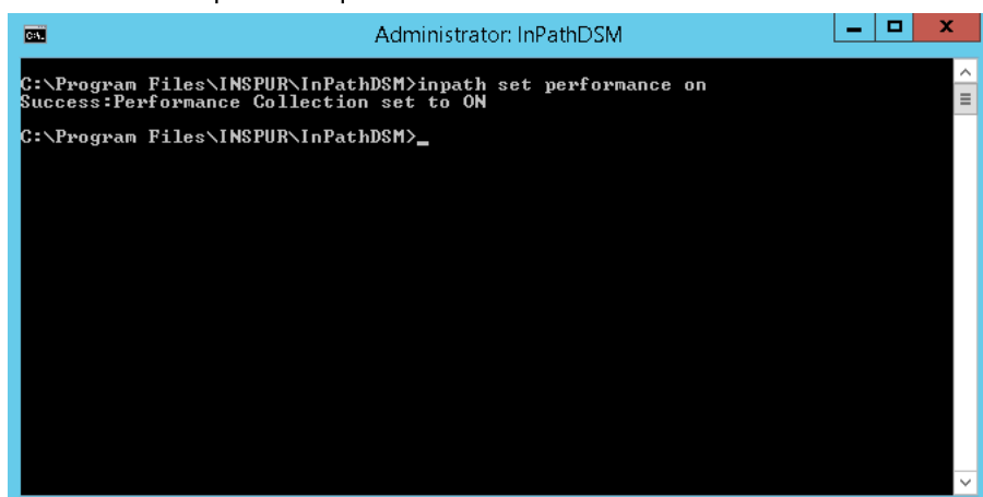
图 4-20 执行 inpath set performance on 命令
